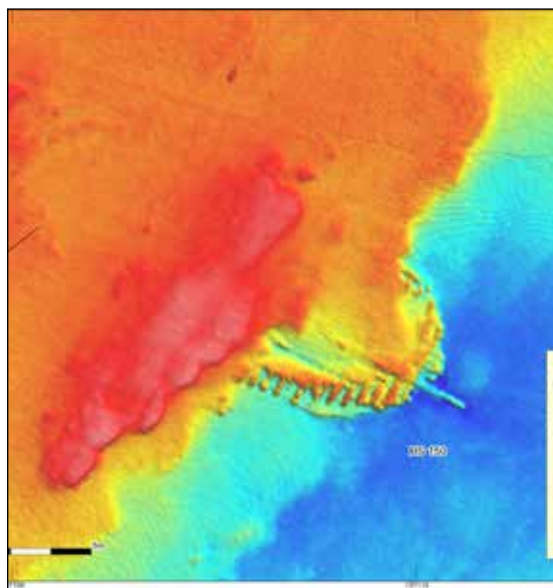
Sonarscan van een historisch scheepswrak nabij Wijdenes. Het wrak steekt uit de modder.
